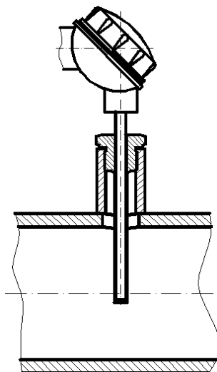
Рисунок 13— Вертикальная установка термометра сопротивления
