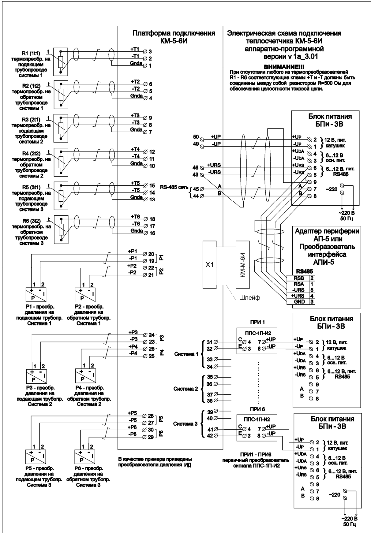
Рисунок Л.2 — Базовая электрическая схема подключения КМ-5-БИ к блокам питания и периферийным устройствам при использовании в качестве преобразователей объема приборов ППС-1П-I2
