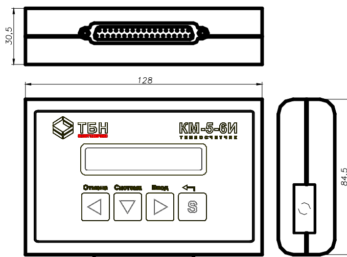
Рисунок 5 — Внешний вид, габаритные размеры КМ-М-6И
