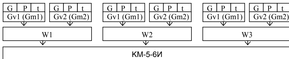
Рисунок 1— Структурная схема теплосчётчика КМ-5-6И
